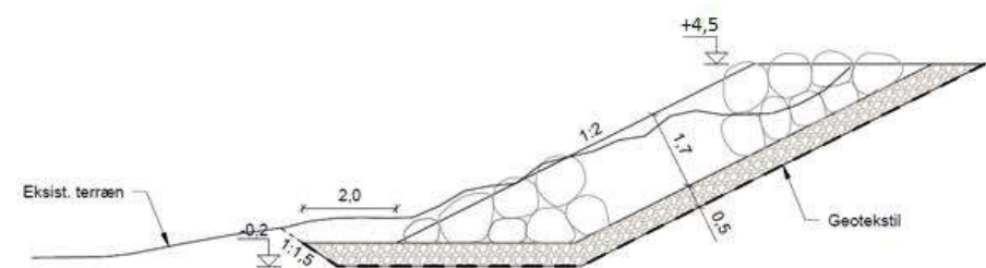
PRINCIPSNIT , 1:100 Strækning B
