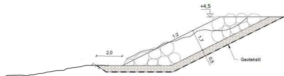
PRINCIPSNIT, 1:100 Strækning B
